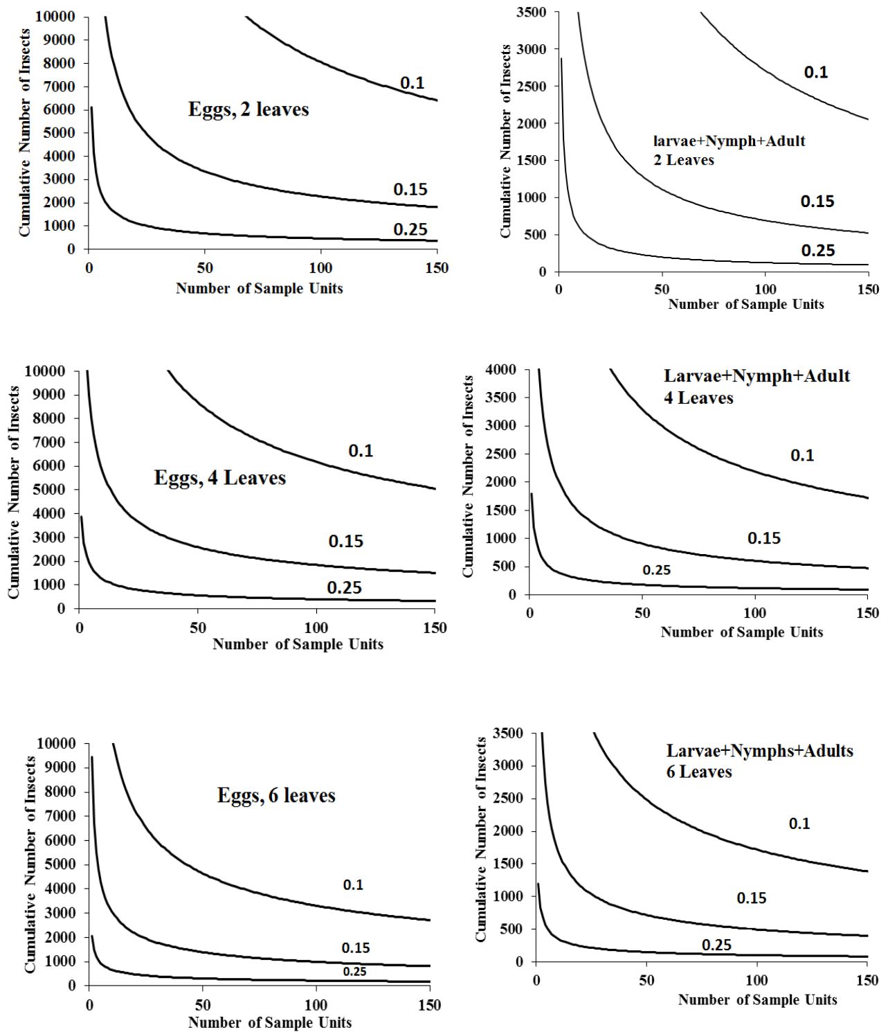
شکل ۱- خطوط توقف در نمونه‌گیری دنباله‌ای با دقت ثابت به روش گرین در واحدهای نمونه دو، چهار و شش برگ به منظور تخمین تراکم جمعیت کنه تارتن دولک‌های Tetranychus urticae در مزارع لوبیا قرمز با سه سطح خطای ۰/۱، ۰/۱۵ و ۰/۲۵
